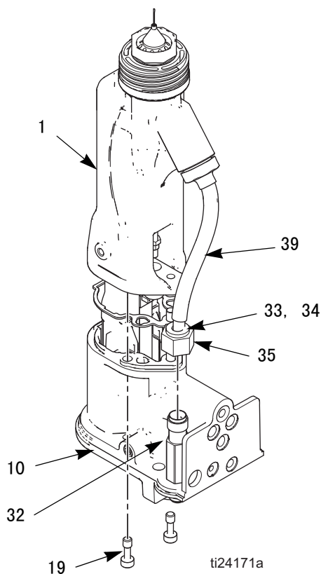
图 24. 枪管拆卸
