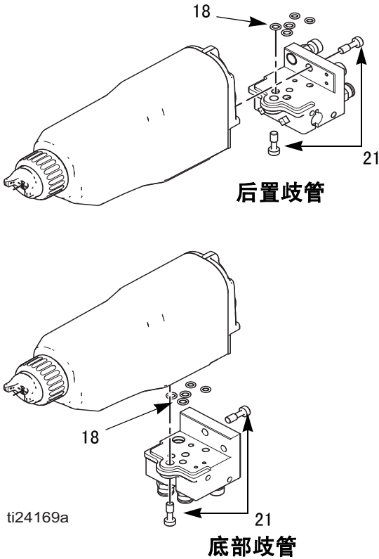
图 17. 从歧管上卸下喷枪
