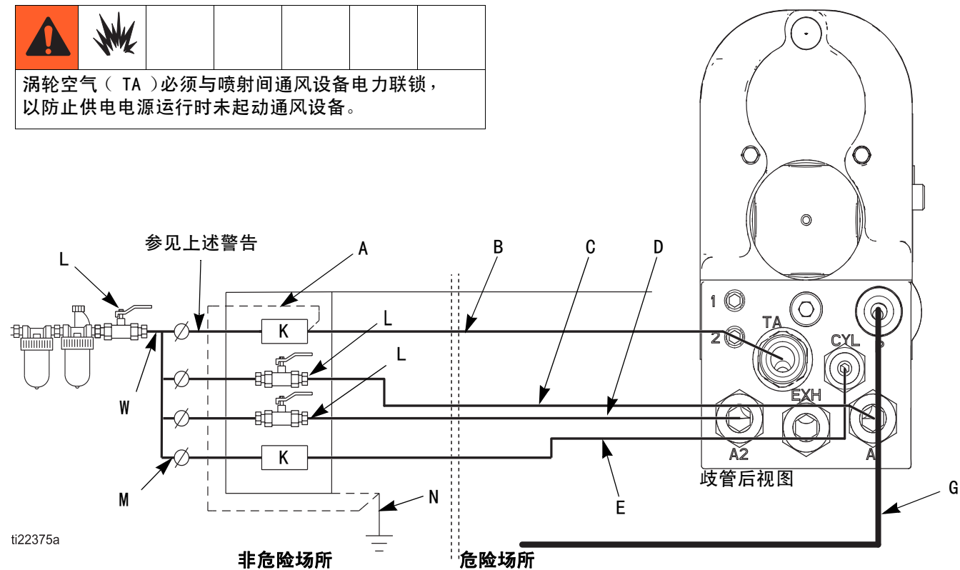
图 3. 典型安装
