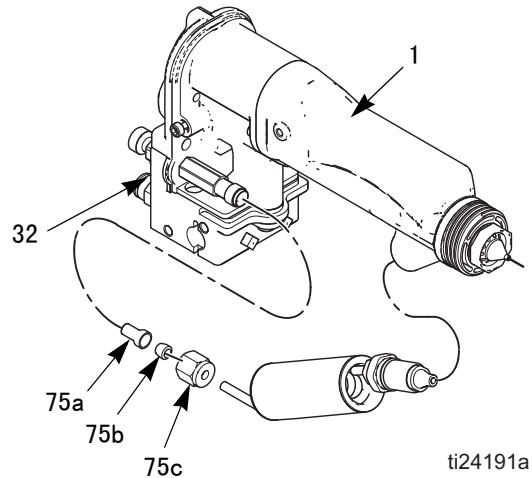
图 10. 高导电率转换配件包
