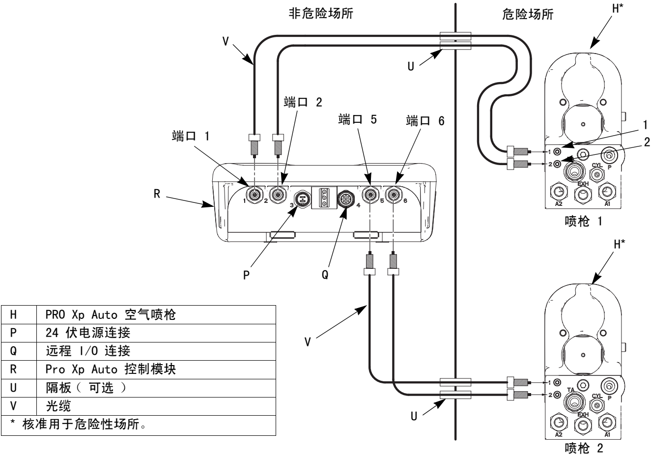
图 7. 光纤原理图
