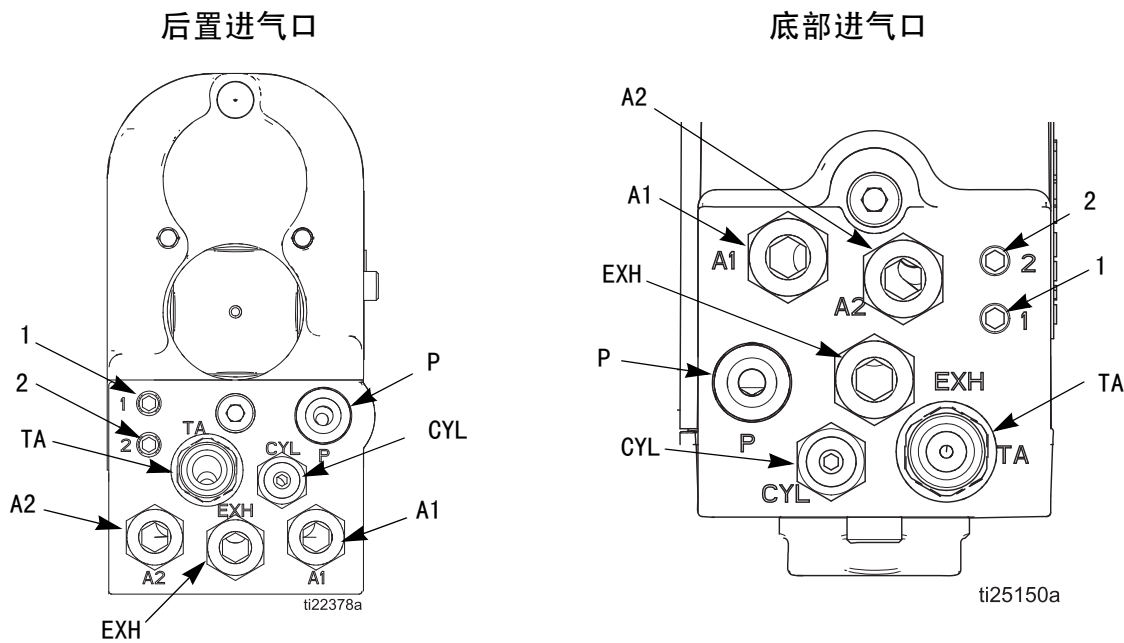
图 5. 歧管连接
