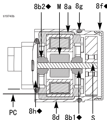
图 29. 涡轮横截面
