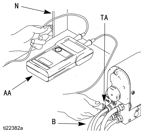
图 8. 检查喷枪的接地
