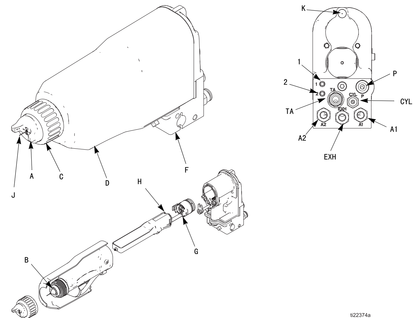
图 2. 喷枪概述
