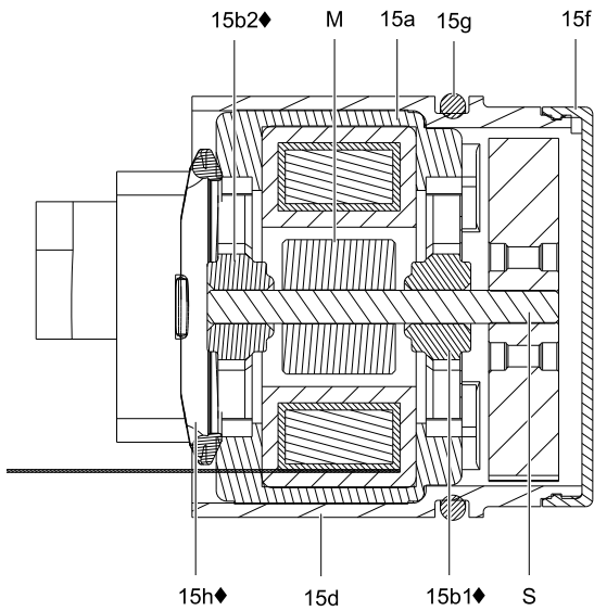
Figure 29 交流发电机横截面
