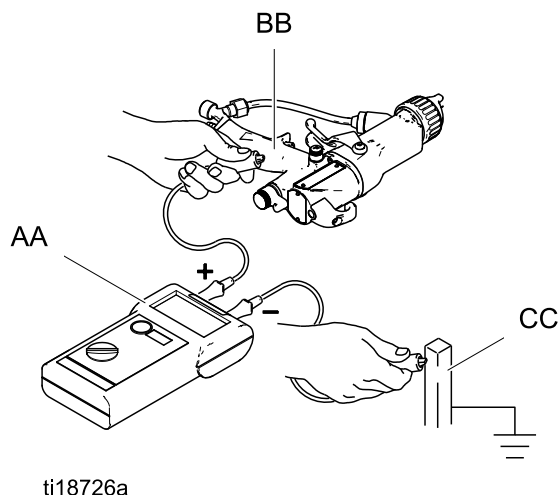
Figure 16 检查喷枪电气接地
