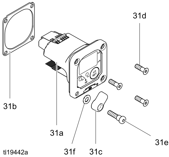
部件号 24N756 智能模块组件
