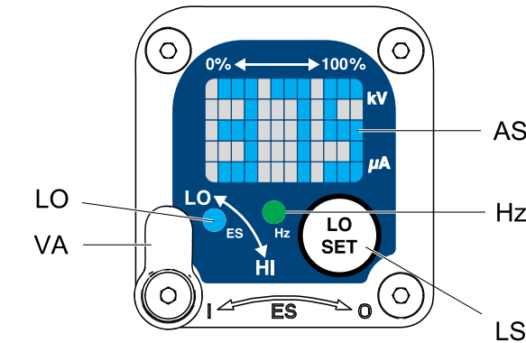
ti19125a Figure 8 交流发电机速度（赫兹）屏幕
