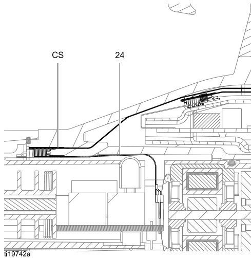
Figure 27 连接柔性电路
