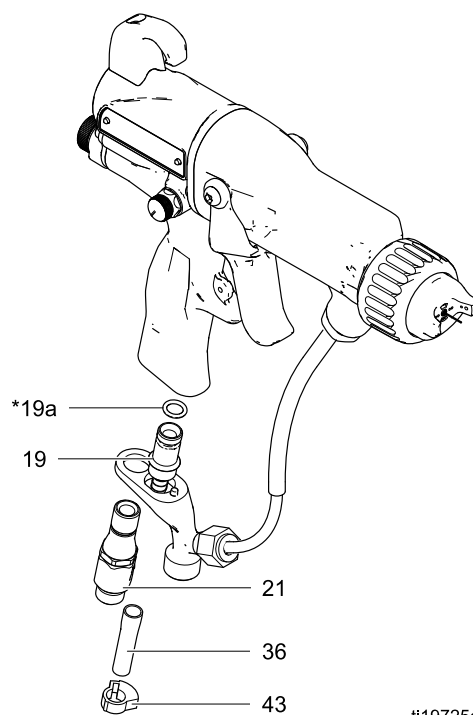
Figure 37 空气入口管接头和排气阀
